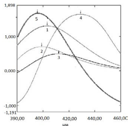
Рис. 1. УФ-спектры водно-этанольного извлечения из сбора (1), СО лютеолина (2), СО рутина (3), СО кверцетина (4), водного извлечения из сбора (5)
