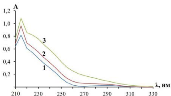
Рис. 2. Зависимость оптической плотности растворов молекулярной формы кетоконазола ( \text{pH}=13 ) от длины волны. 1 – C(\text{кет})=2,5 \cdot 10^{-5} моль/л; 2 – C(\text{кет})=2,5 \cdot 10^{-5} моль/л, C(\text{тиз})=1,0 \cdot 10^{-5} моль/л; 3 – C(\text{кет})=1,0 \cdot 10^{-5} моль/л, C(\text{тиз})=5,0 \cdot 10^{-5} моль/л
